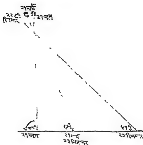
चित्र सख्या ५६—डलाहाबाद में मध्याह्न के समय सूर्य की ऊँचाई
